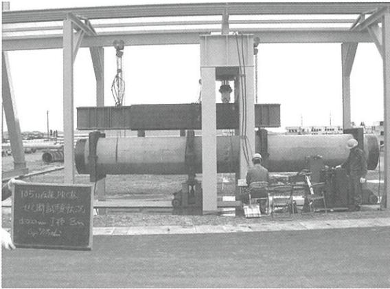
φ 1000mm（Ⅰ種）せん断実験の全景
